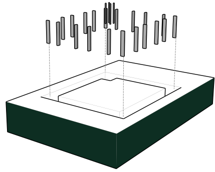
Temel demir donatılarına kaynaklanan çelik lamalar yerleştirilir.
