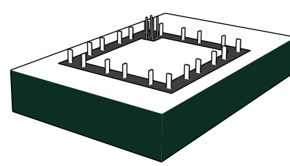
Betonun prizini almasından sonra boşluk toprak ile doldurulur ve sıkıştırılır.
