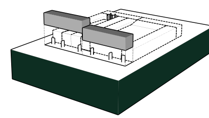
Aynı eksenle atölye ortamında delikleri açılan taş bloklar epoksi yapıştırıcı uygulandıktan sonra yerlerine yerleştirilir.
