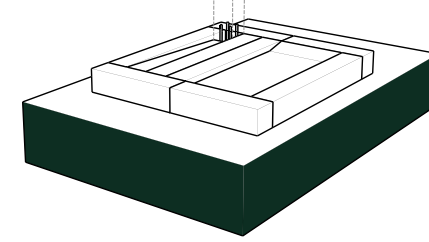
Tüm yatay taşların yerlerine yerleştirilmesinden sonra dikey taş eleman yerine aynı teknikle yerleştirilir.
