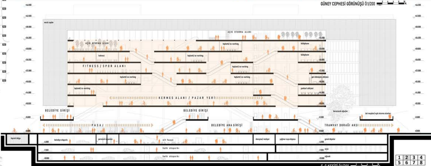
C-C KESİTİ 0:1/200
