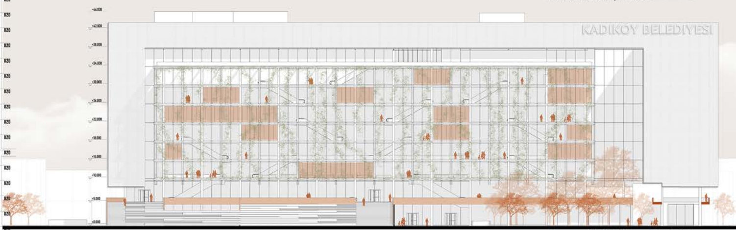
GÜNEY CEPHESİ GÖRÜNÜŞÜ 0:1/200
